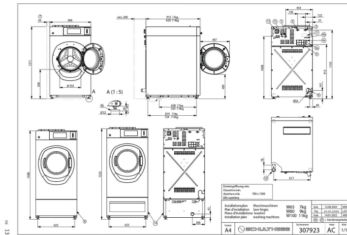
Dimensions
